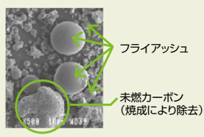
日本製紙(株)石巻工場のフライアッシュ(焼成前)電子顕微鏡写真
