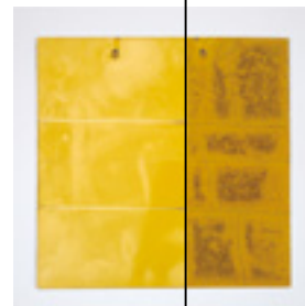
設置:垂直 屋外7年 左側:施工済 / 右側:未施工
